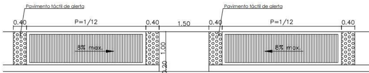
Rampa paralela
